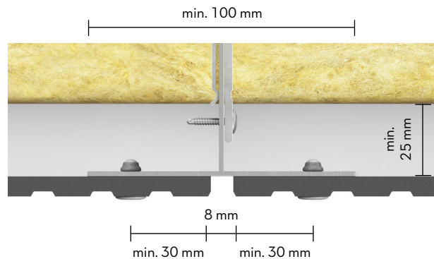
Rys. 1. Montaż Cembrít Patina Inline na profilu „T”
