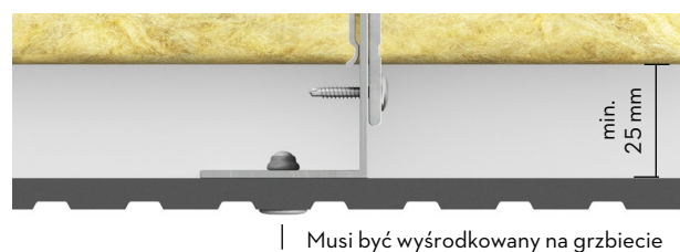
Rys. 2. Montaż Cembrít Patina Inline na profilu „L”
