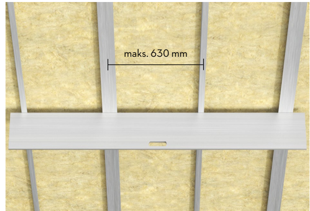
Prostoliniowość podkonstrukcji
