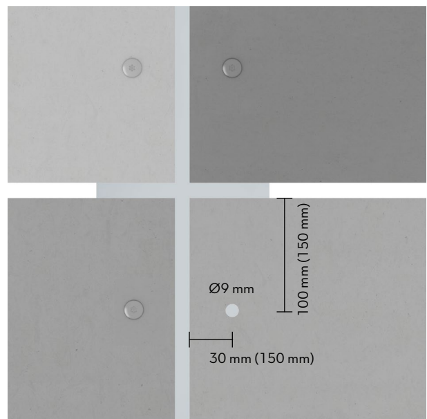
Przykład podkonstrukcji pionowej
