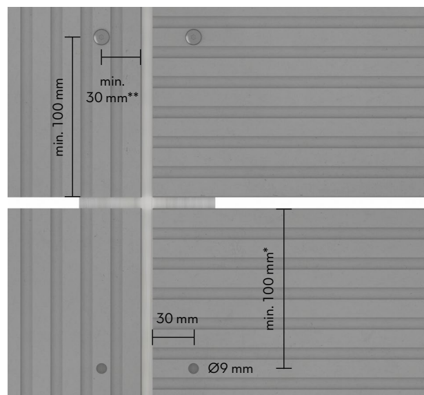
Rys. 3. Odległości między krawędziami Cembrít Patina Inline Uwaga! Minimalna odległość i/lub najbliższy następny grzbiet
