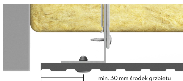
Rys. 4. Montaż Cembrít Patina Inline na płycie przyciętej na wymiar
