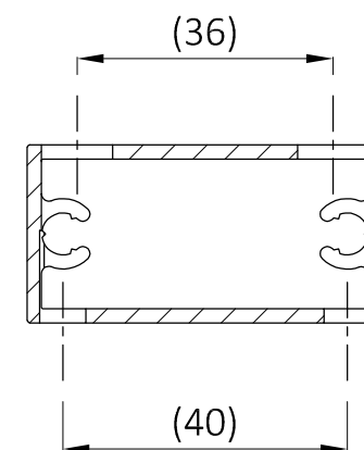
PRZEKRÓJ A-A
